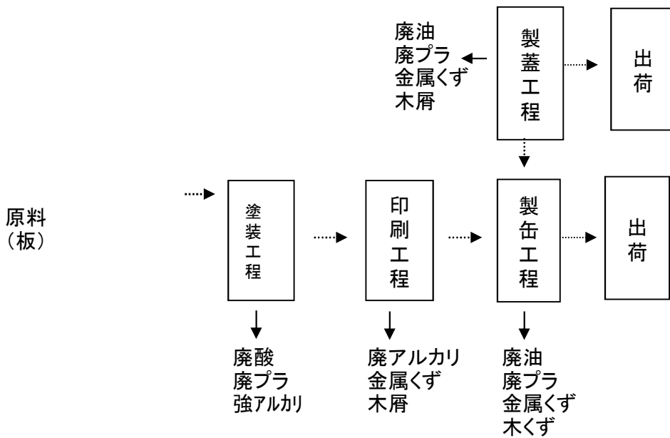
図-2 飲料缶(印刷)・粉乳缶製造フローシート
