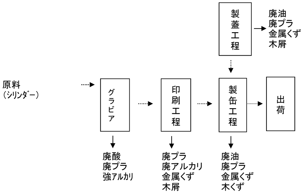
図-1 飲料缶(クリスタル缶)製造フローシート
