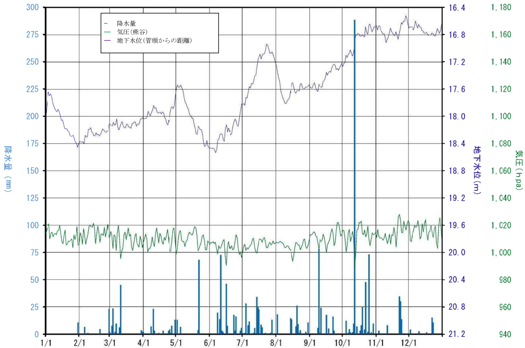
図-2.1.2 浦和東観測所 地下水位変動図
